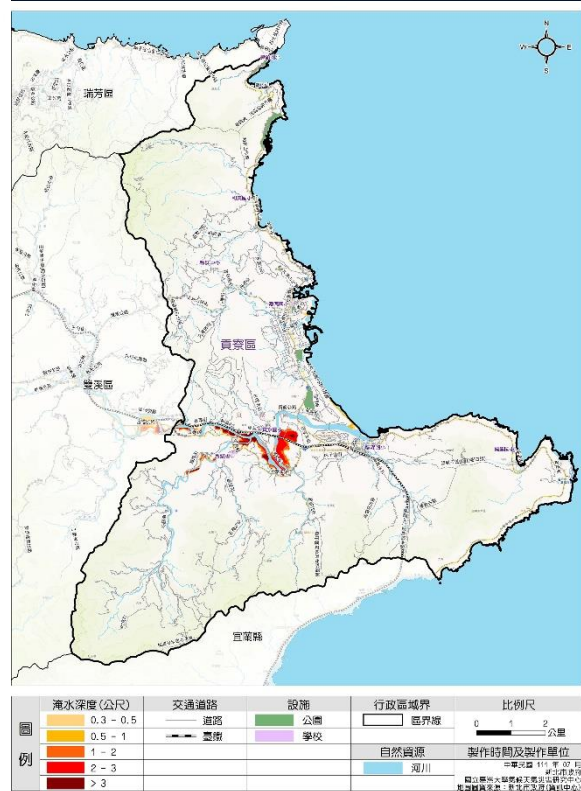
新北市貢寮區24小時累積雨量500毫米淹水潛勢圖
