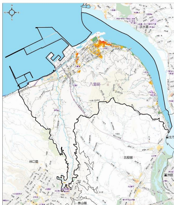
新北市八里區24小時累積雨量500毫米淹水潛勢圖
