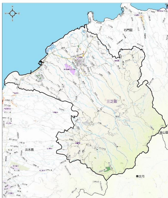
新北市三芝區24小時累積雨量500毫米淹水潛勢圖
