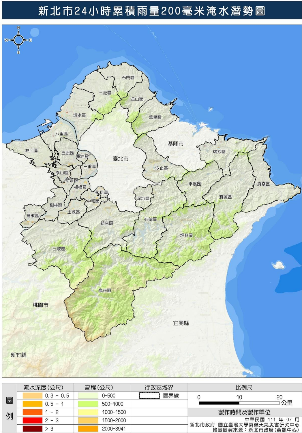
新北市淹水潛勢圖(24 小時延時 200 毫米/天)
