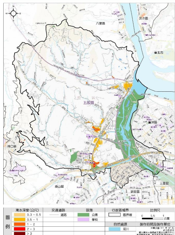
新北市五股區24小時累積雨量500毫米淹水潛勢圖
