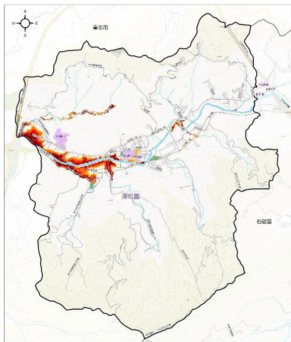
新北市深坑區24小時累積雨量500毫米淹水潛勢圖
