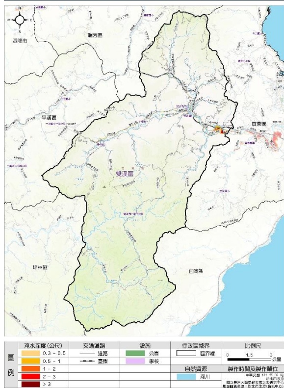
新 北 市 雙 溪 區 24 小 時 累 積 雨 量 500 毫 米 淹 水 潛 勢 圖
