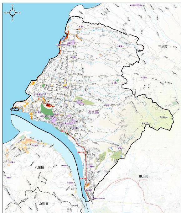
新北市淡水區24小時累積雨量500毫米淹水潛勢圖
