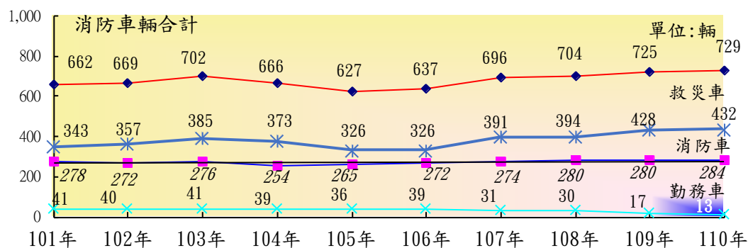
圖3.1、新北市101年至110年各式消防車輛變遷統計圖
